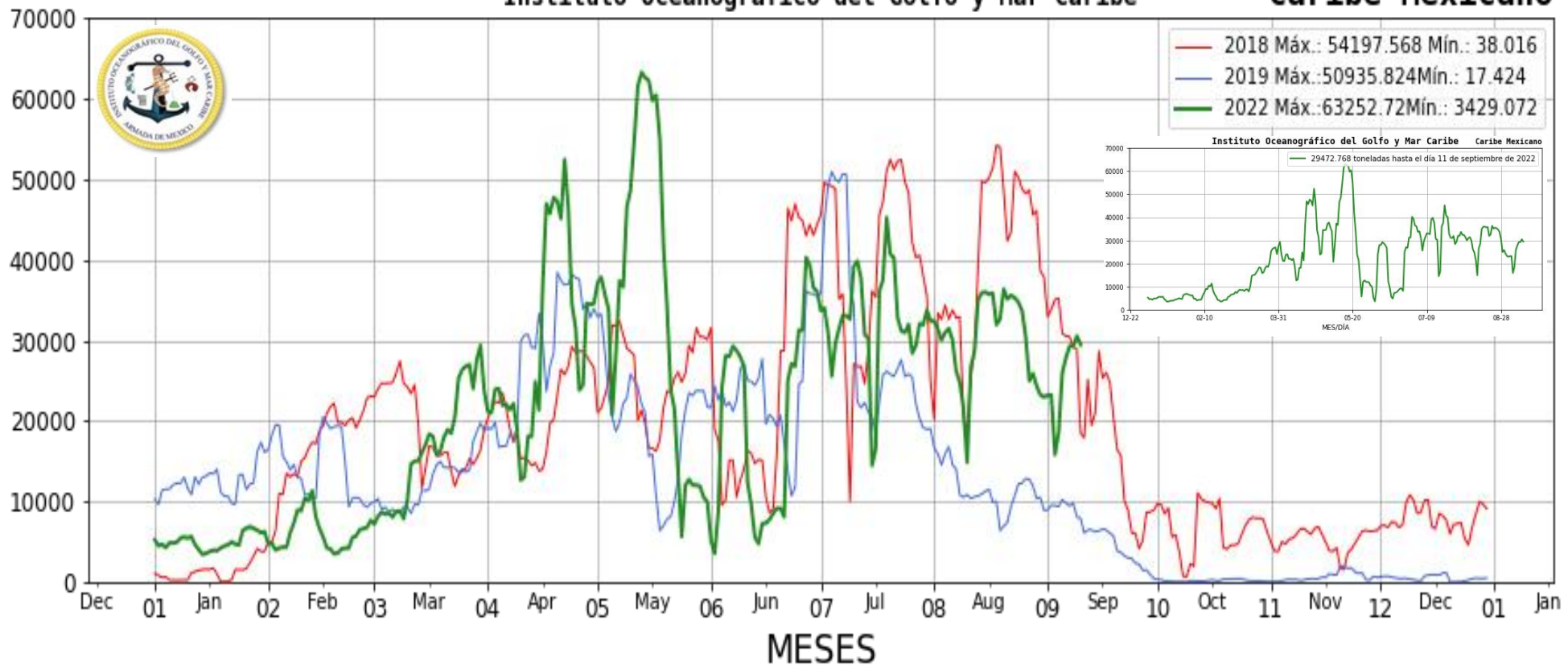
Figura 2.- Valores estimados de la cantidad de sargazo en el Caribe Mexicano. Gráfico comparativo de los años 2018, 2019 y 2022 (gráfico mayor) y valores estimados del 01 de enero al 11 de septiembre del presente año (gráfico superior derecha) obtenidos a partir de datos de la USF.
