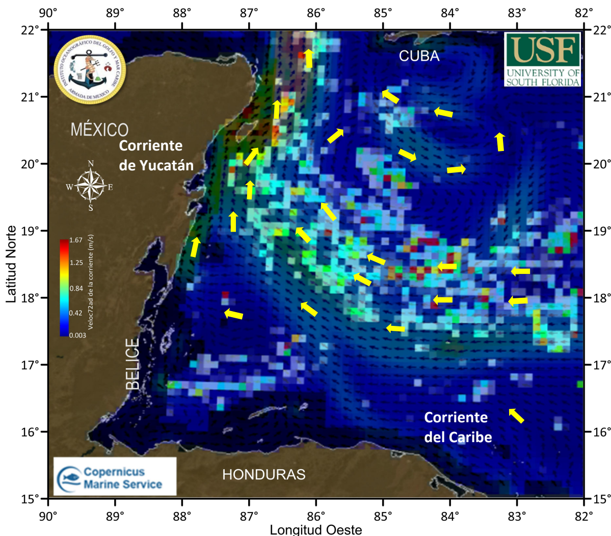
Figura 1.- Cobertura algal (11 de septiembre) y modelación de corrientes superficiales (12 de septiembre).
