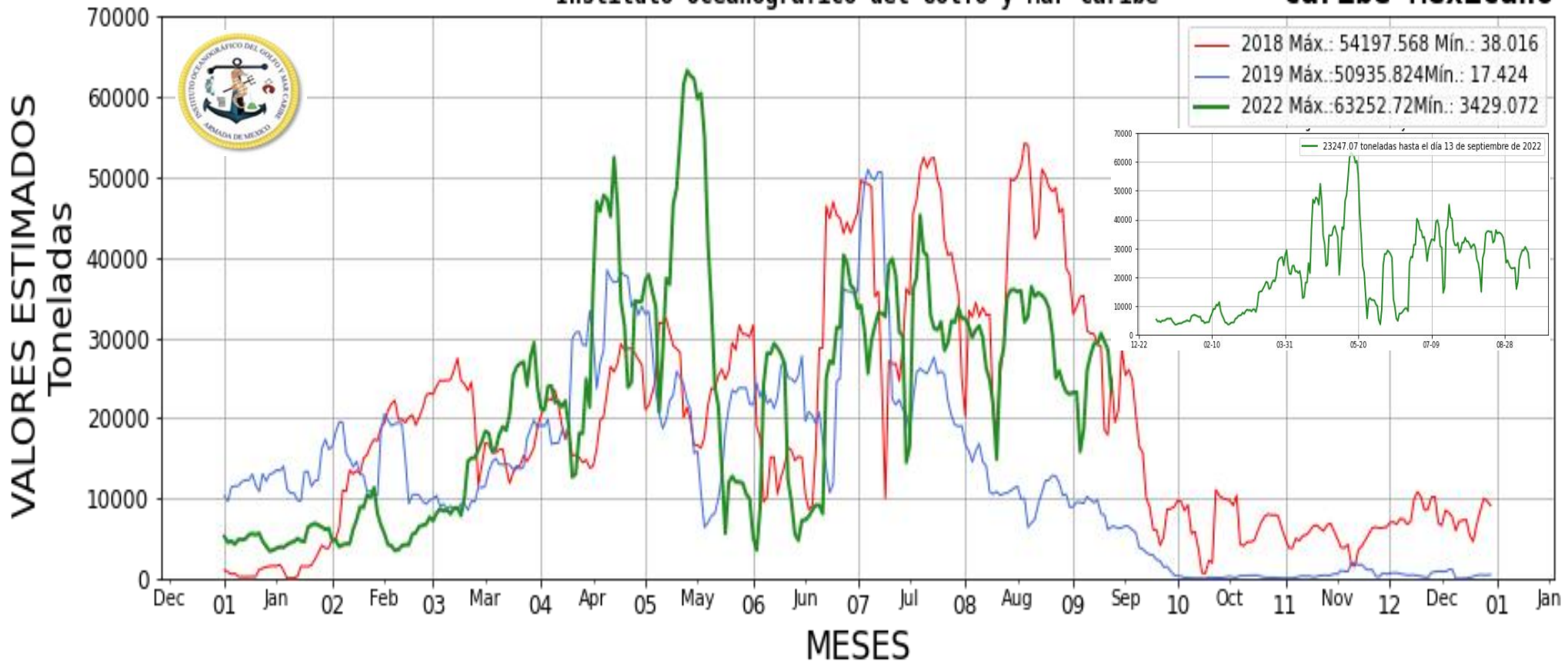
Figura 2.- Valores estimados de la cantidad de sargazo en el Caribe Mexicano. Gráfico comparativo de los años 2018, 2019 y 2022 (gráfico mayor) y valores estimados del 01 de enero al 13 de septiembre del presente año (gráfico superior derecha) obtenidos a partir de datos de la USF.
