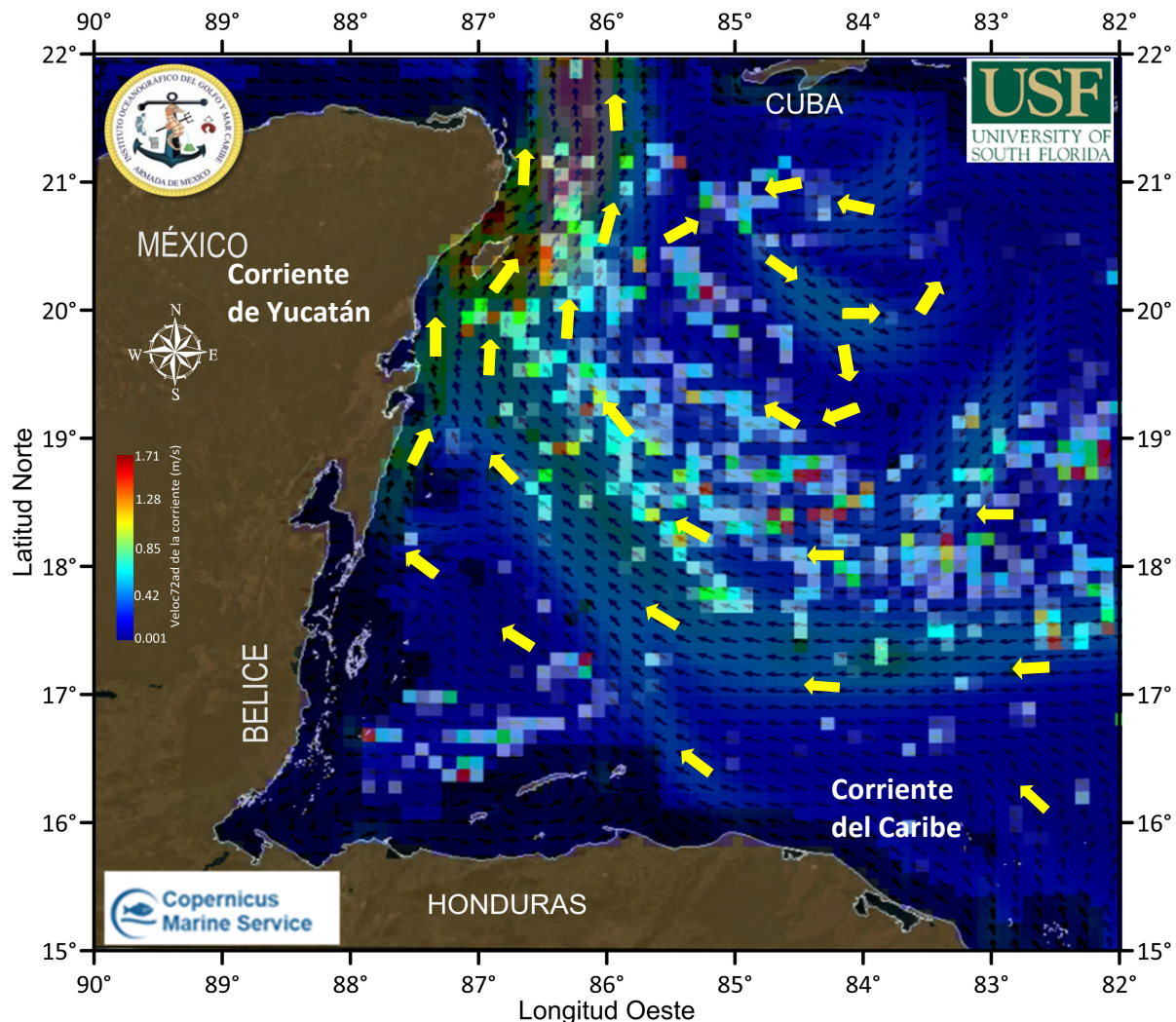
Figura 1.- Cobertura algal (13 de septiembre) y modelación de corrientes superficiales (14 de septiembre).
