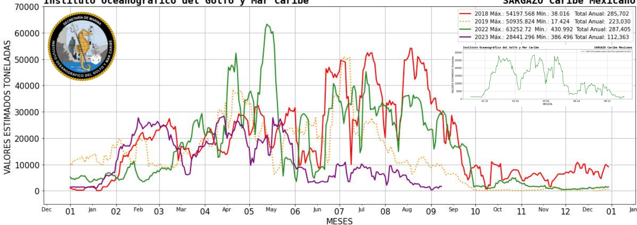
Figura 2.- Presencia aproximada de sargazo en el Caribe Mexicano. Gráfico comparativo de los años 2018, 2019, 2022 y 2023 (gráfico mayor) y valores estimados del 01 de enero al 09 de septiembre del presente año (gráfico superior derecho) obtenidos a partir de datos de la USF.
