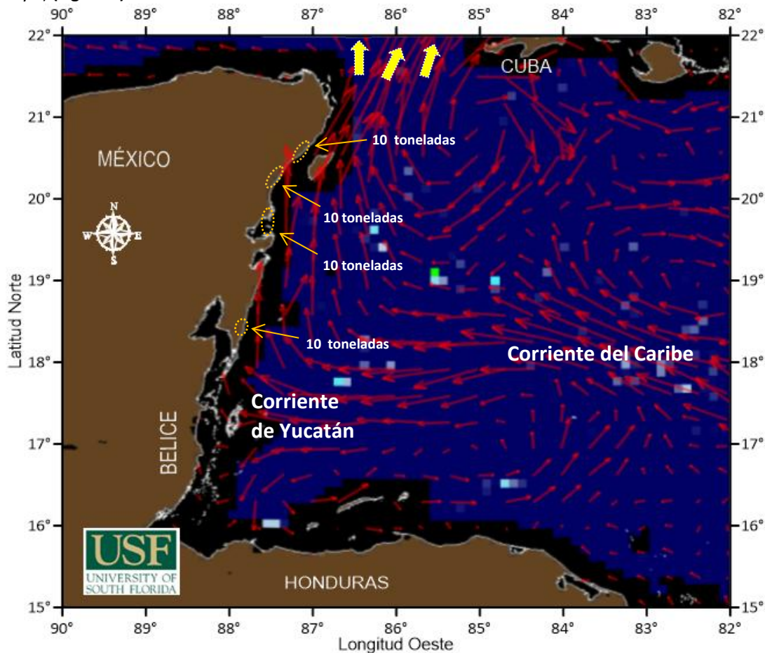
Figura 1.- Cobertura algal (08 de septiembre) y la modelación de corrientes superficiales (09 de septiembre), obtenidos a partir de datos de la USF.
