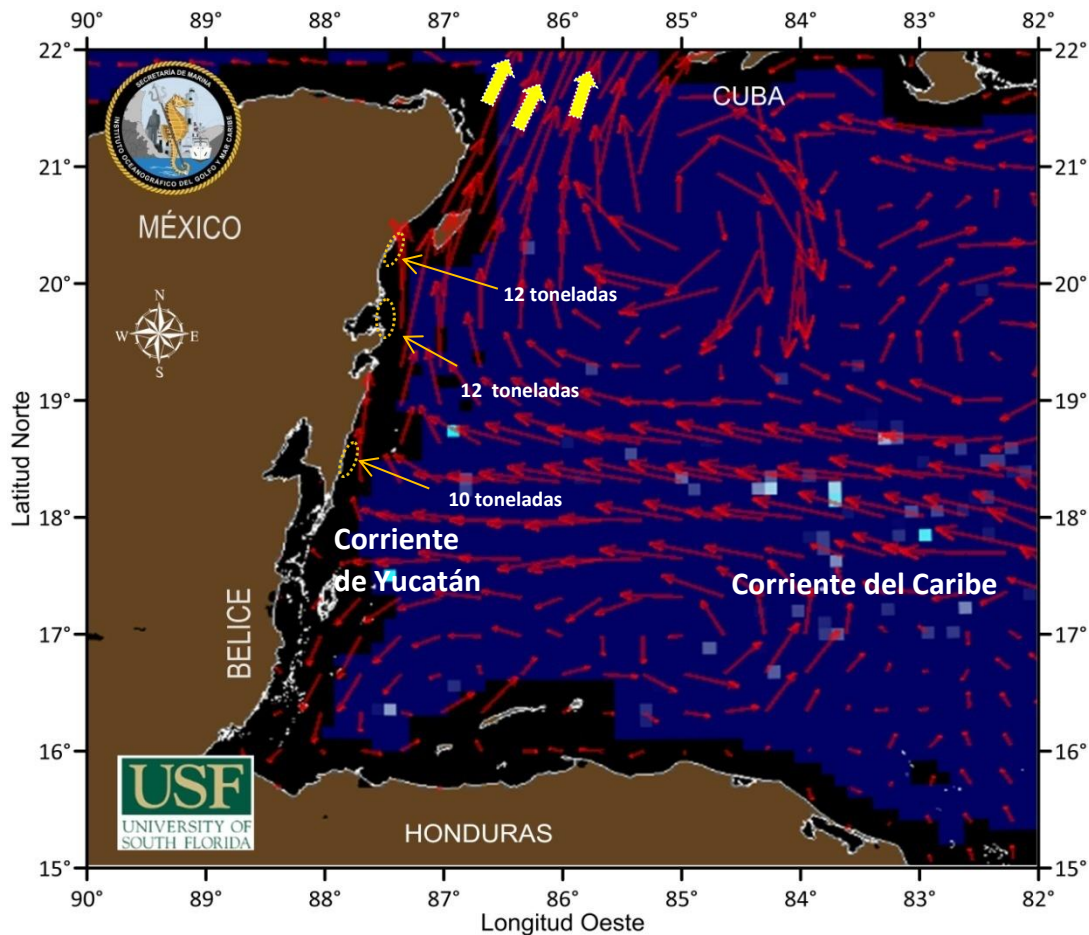
Figura 1.- Cobertura algal (16 de septiembre) y la modelación de corrientes superficiales (17 de septiembre), obtenidos a partir de datos de la USF.
