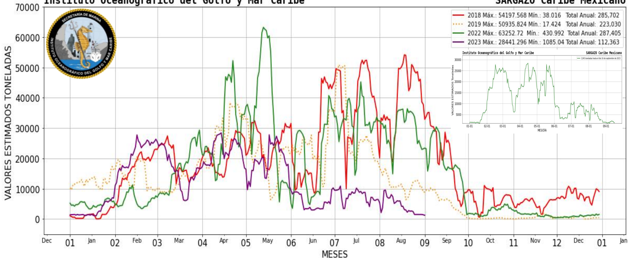
Figura 2.- Presencia aproximada de sargazo en el Caribe Mexicano. Gráfico comparativo de los años 2018, 2019, 2022 y 2023 (gráfico mayor) y valores estimados del 01 de enero al 16 de septiembre del presente año (gráfico superior derecho) obtenidos a partir de datos de la USF.
