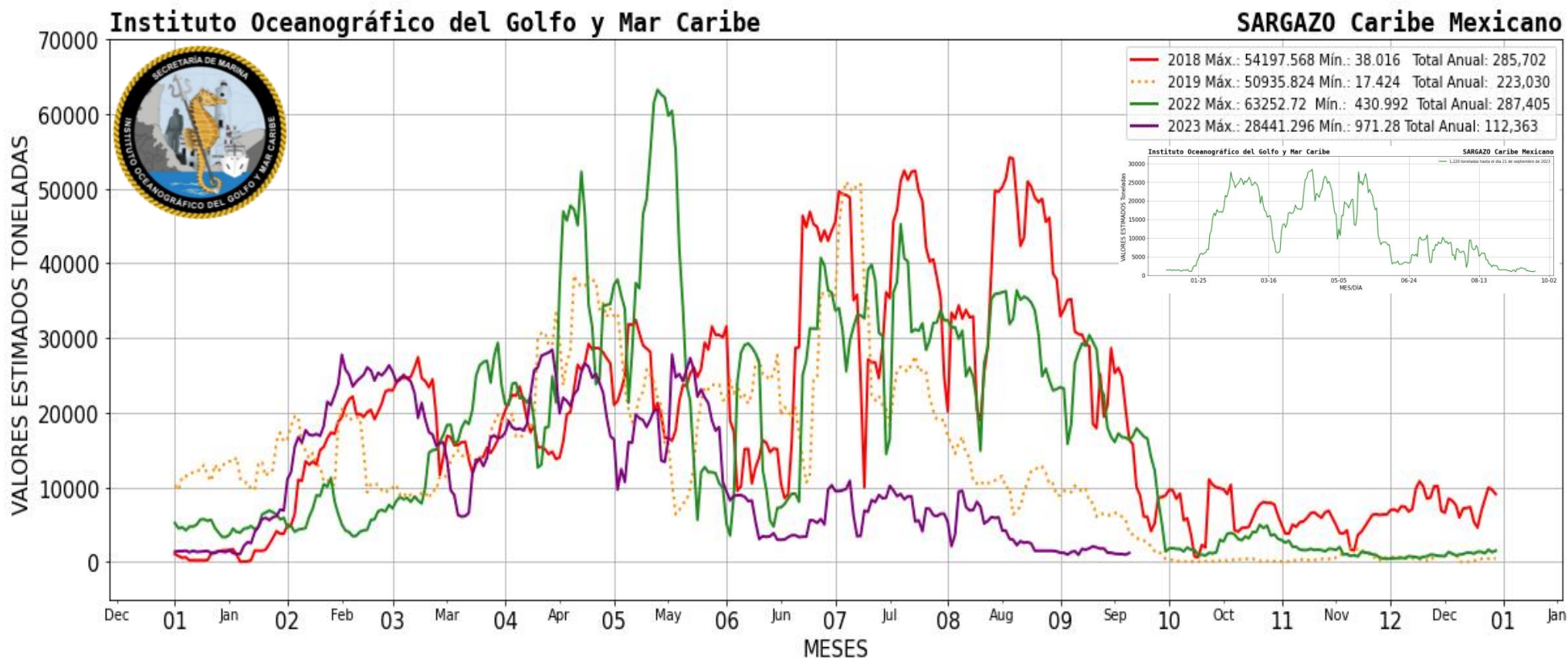
Figura 2.- Presencia aproximada de sargazo en el Caribe Mexicano. Gráfico comparativo de los años 2018, 2019, 2022 y 2023 (gráfico mayor) y valores estimados del 01 de enero al 21 de septiembre del presente año (gráfico superior derecho) obtenidos a partir de datos de la USF.
