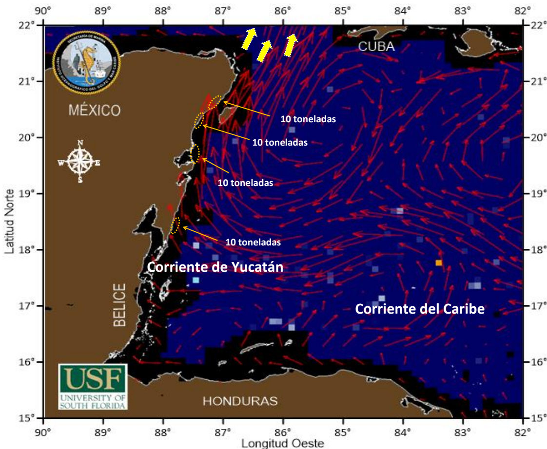
Figura 1.- Cobertura algal (21 de septiembre) y la modelación de corrientes superficiales (22 de septiembre), obtenidos a partir de datos de la USF.
