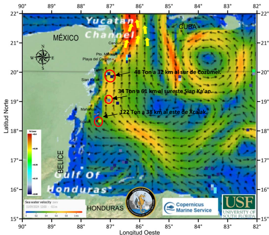
Figura 2.- Cobertura algal ( 14 de septiembre ) y la modelación de corrientes superficiales ( 15 de septiembre ), obtenidos a partir de datos de la USF.
