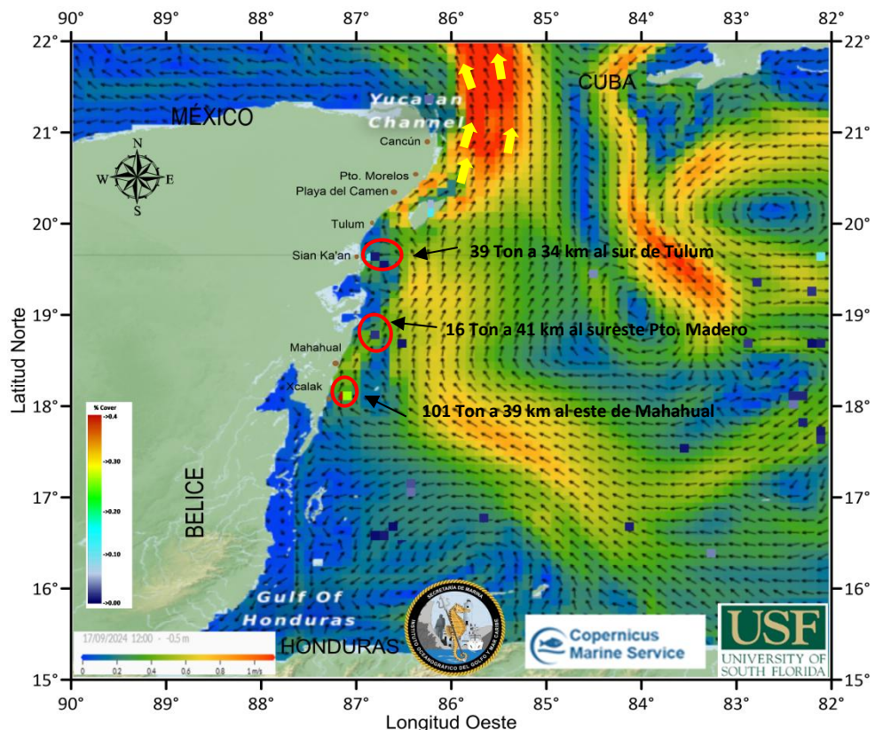
Figura 2.- Cobertura algal (16 de septiembre) y la modelación de corrientes superficiales (17 de septiembre), obtenidos a partir de datos de la USF.
