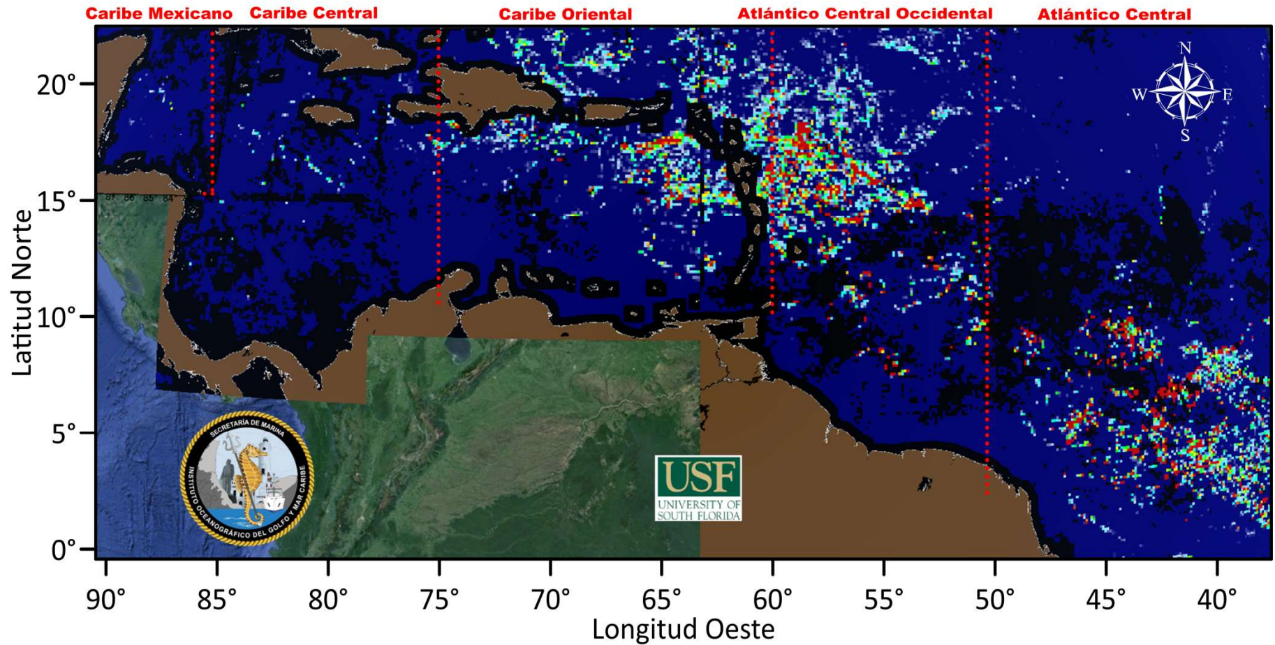
Figura 1.- Cobertura algal (16 de junio de 2024) para las distintas regiones del Atlántico y Mar Caribe, a partir de datos de la USF.
