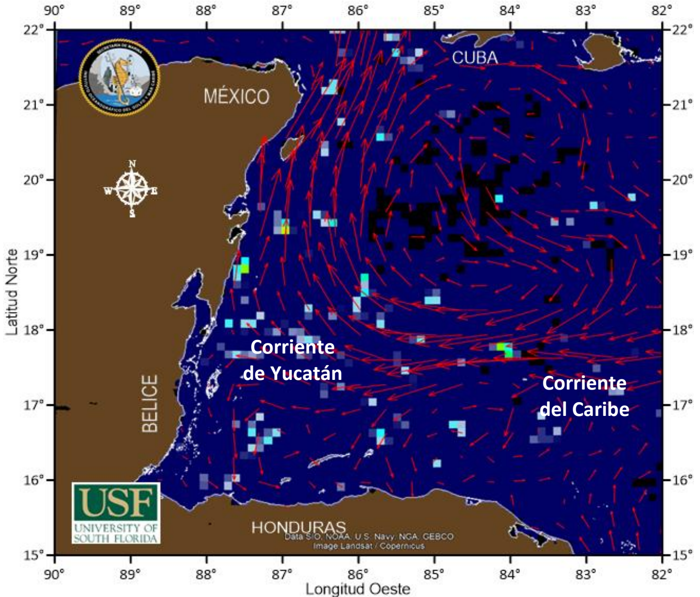
Figura 1.- Cobertura algal (19 de marzo) y la modelación de corrientes superficiales (20 de marzo).
