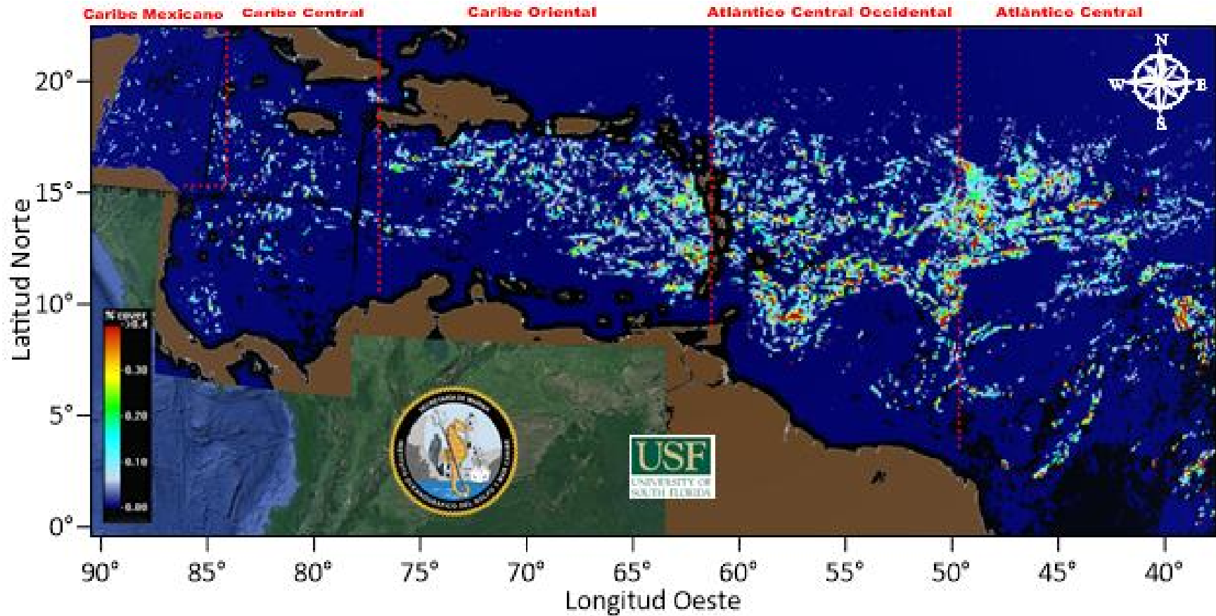
Figura 2.- Densidad de algas flotantes (FA) en términos de porcentaje de cobertura, por regiones, según USF-OOL. Imágenes del día 19 de marzo.
