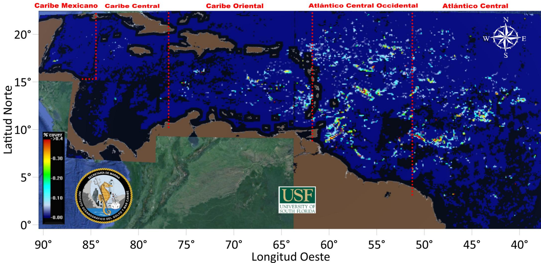
Figura 1.- Cobertura algal (21 de marzo de 2024) para las distintas regiones del Atlántico y Mar Caribe, a partir de datos de la USF.
