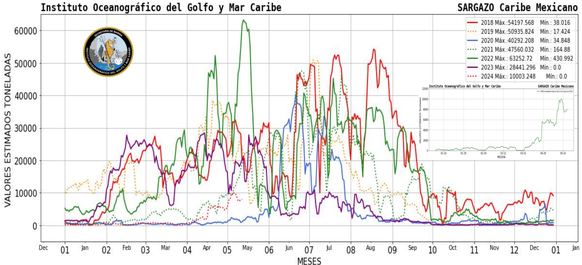
Figura 3.- Densidad de sargazo calculada como una media de los 7 días anteriores (incluido el día actual), basada en las imágenes correspondientes del Índice Alternativo de Algas Flotantes (AFAI) utilizando el método descrito en Wang y Hu (2016). Gráfico comparativo de los años 2018-2024 (gráfico mayor) y valores estimados del 01 de enero al 12 de mayo del presente año (gráfico superior derecho) obtenidos a partir de datos de la USF.
