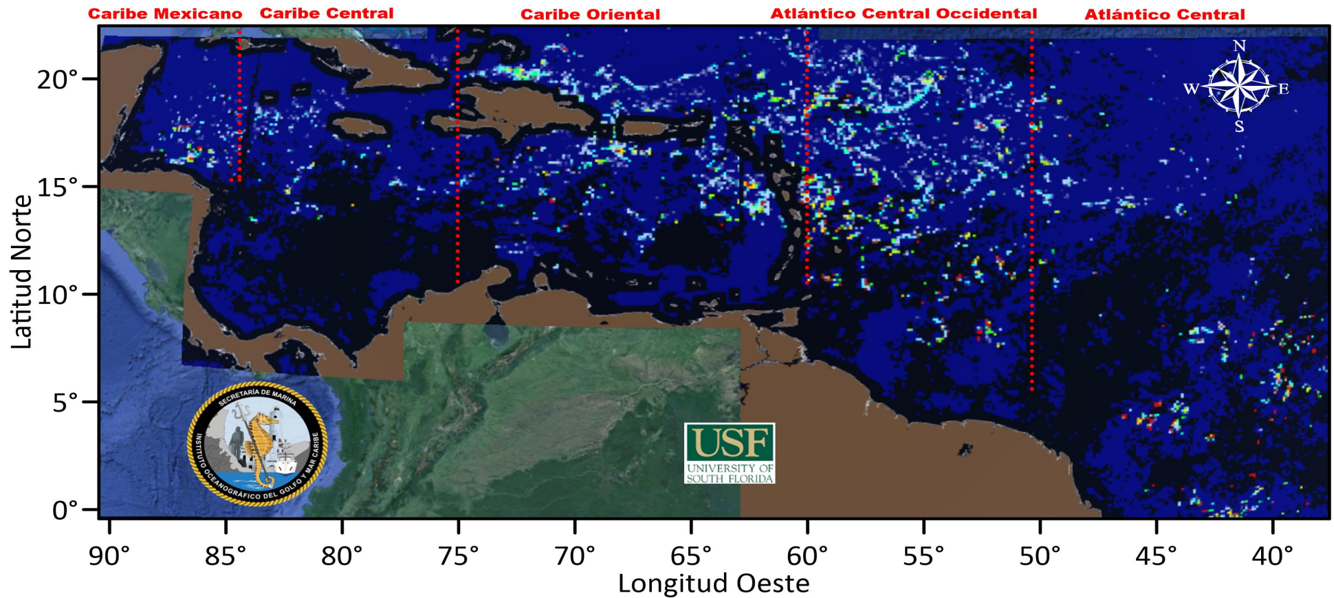
Figura 1.- Cobertura algal (12 de mayo de 2024) para las distintas regiones del Atlántico y Mar Caribe, a partir de datos de la USF.
