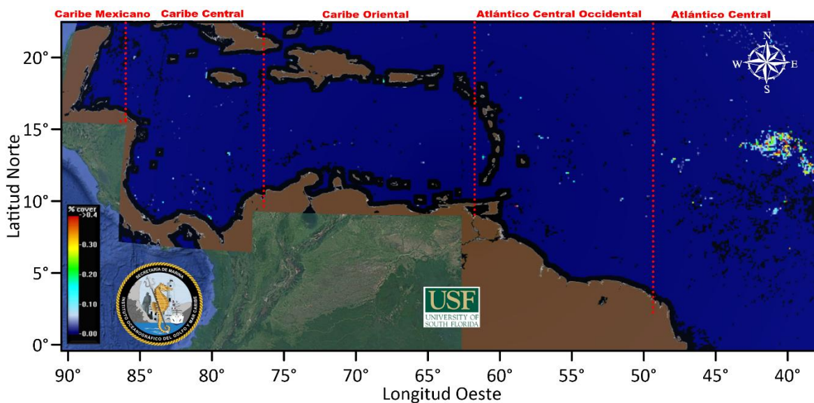
Figura 1.- Cobertura algal (24 de noviembre) para las distintas regiones del Atlántico y Mar Caribe, a partir de datos de la USF.
