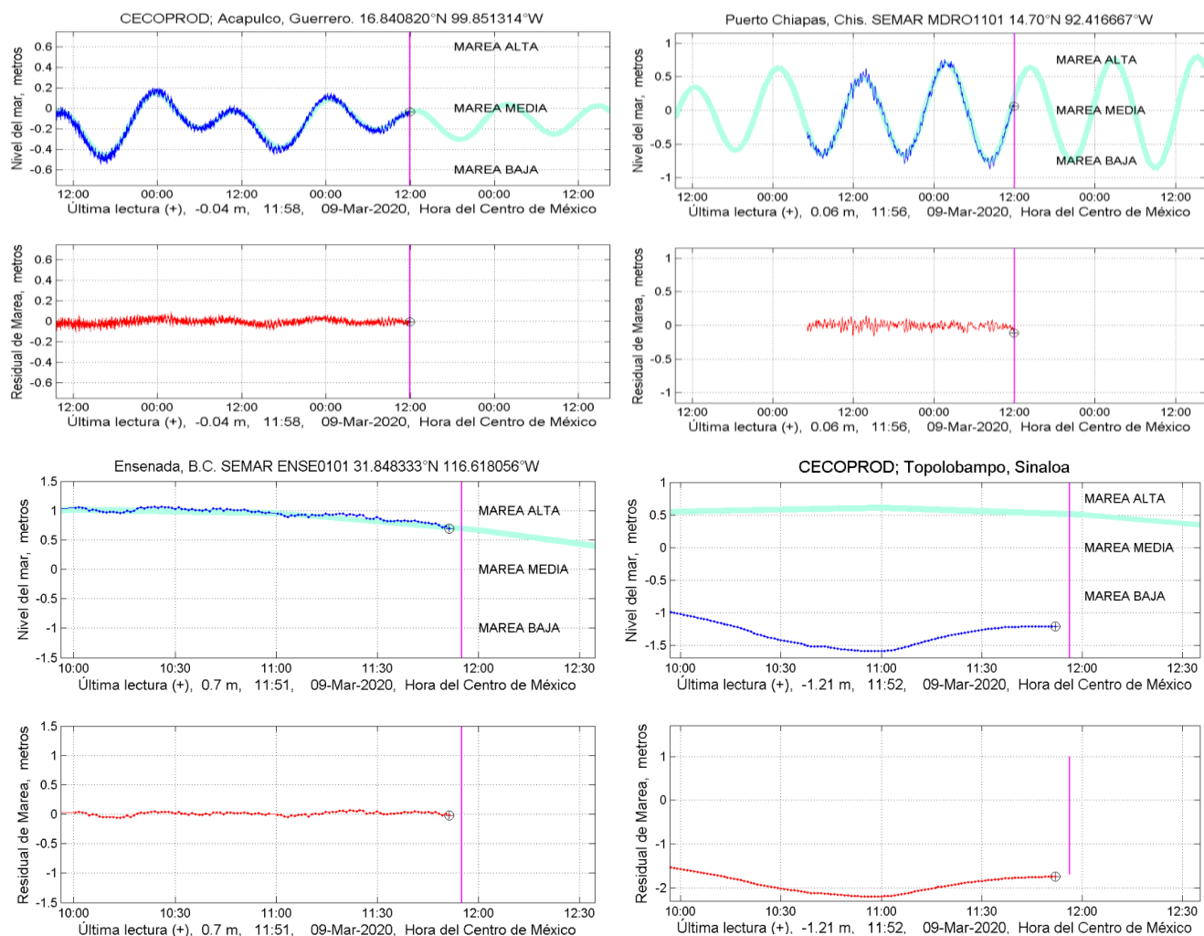
Figura 8. Monitoreo en tiempo real del nivel del mar, provisto por las estaciones mareográficas existentes de la SEMAR al Centro de Alerta de Tsunamis, con el fin de cumplir con los objetivos fundamentales del SINAT.
