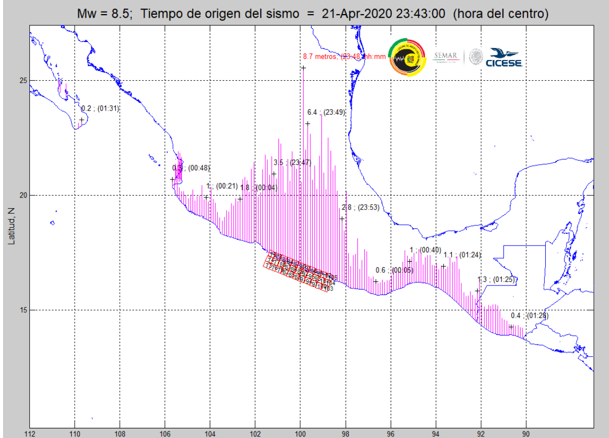
Figura 16. Altura de la ola y hora estimada de arribo de un tsunami por un sismo hipotético magnitud 8.5 en las costas del estado de Guerrero.
